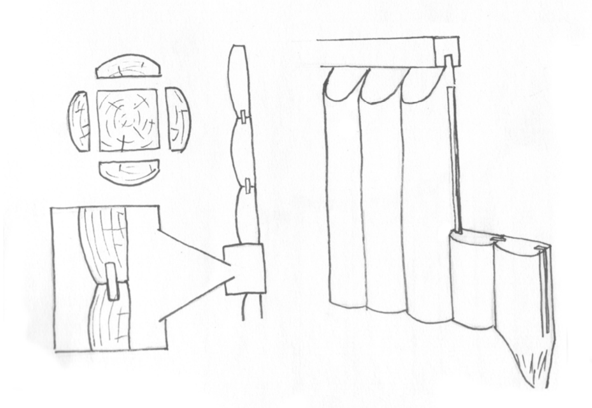
Fig. 1 Palissadväggens konstruktion, baserad på kyrkan i Greensted, samt Eckhoffs rekonstruktion av Hemse. Notera nåtar med lösa fjädrar och hammarband, samt hur stavarna är utkluvna från stocken. Stavarna är lätt spetsade och står i en ränna.
