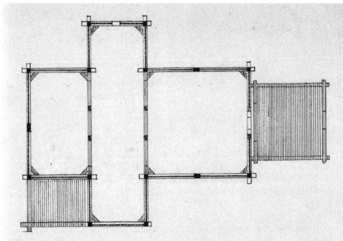
Fortidsminneforeningens plantegning av stavkirken. (De to tilbyggene fra 1700-tallet er nede til venstre og helt til høyre på tegningen).
